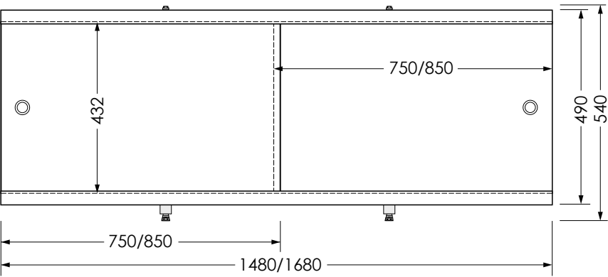
Фронтальный экран. Вид сзади
