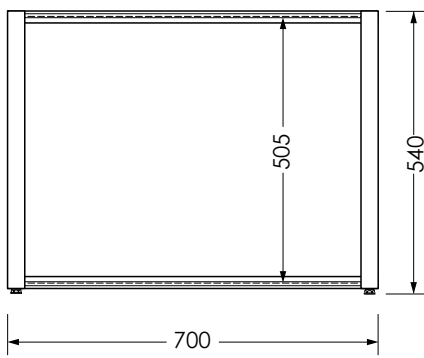
Торцевой экран. Вид спереди
