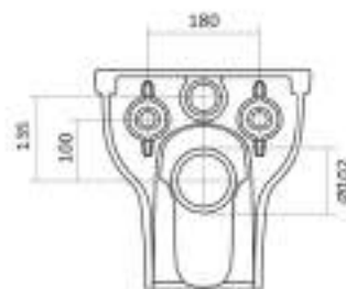
Чаша подвесная безободковая «Лайн rimless» NEW
