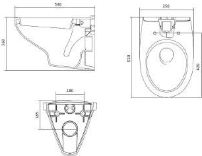
Чаша подвесная «Бореаль»
