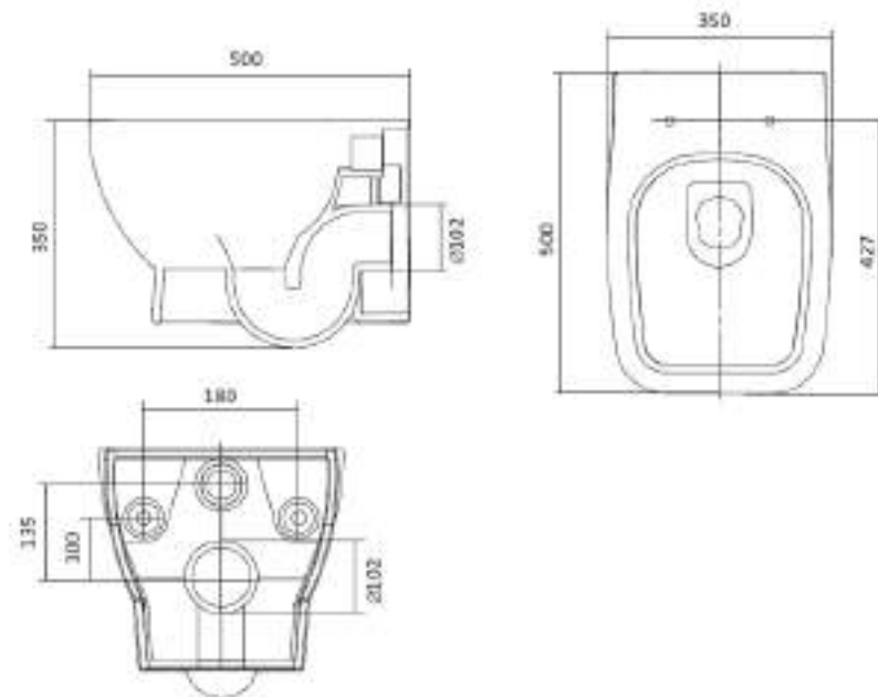
Чаша подвесная «Нео»
