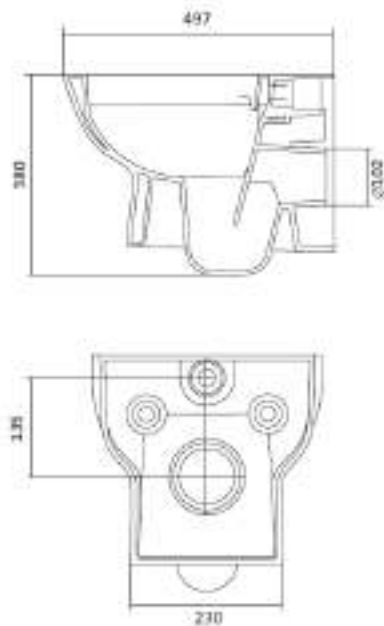
Чаша подвесная безободковая «Neo rimless»
