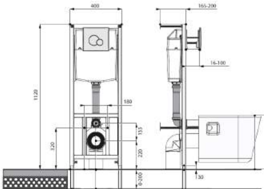
Схема инсталляции для всех комплектов
