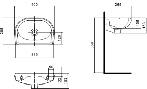
Чертеж умывальника Бриз 40
