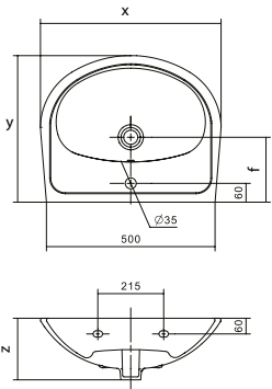
Чертеж умывальников Анимо 50, Анимо 55, Анимо 60
